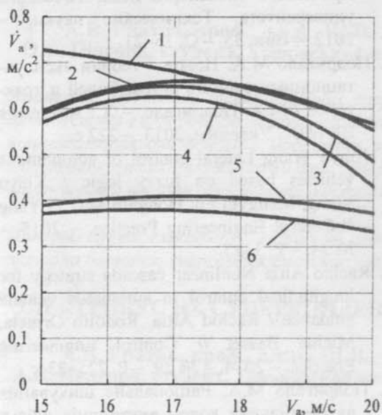
Рис. 5. Графики зависимости ускорения разгона на 5-й передаче автомобилей ГАЗ-3309 с соответствующим пробегом от скорости их движения: 1 – теоретические значения при отсутствии пробега; 2 – пробег 24354 км; 3 – 67234 км; 4 – 105355 км; 5 – 150470 км; 6 – 201232 км
