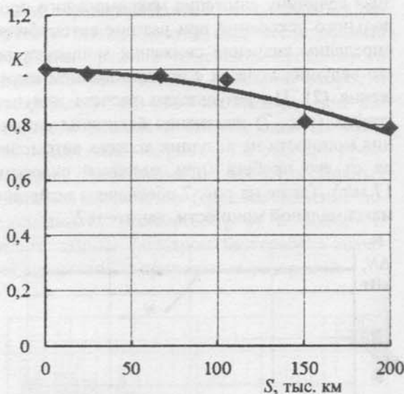
Рис. 8. График изменения коэффициента падения мощности на ведущих колесах автомобилей ГАЗ-3309 от их пробега (скорость движения 17 м/с)
