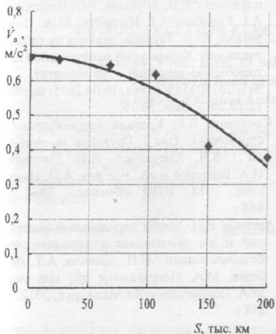
Рис. 6. График изменения максимального ускорения при разгоне на 5-й передаче автомобилей ГАЗ-3309 при увеличении их пробега при скорости движения 17 м/с
