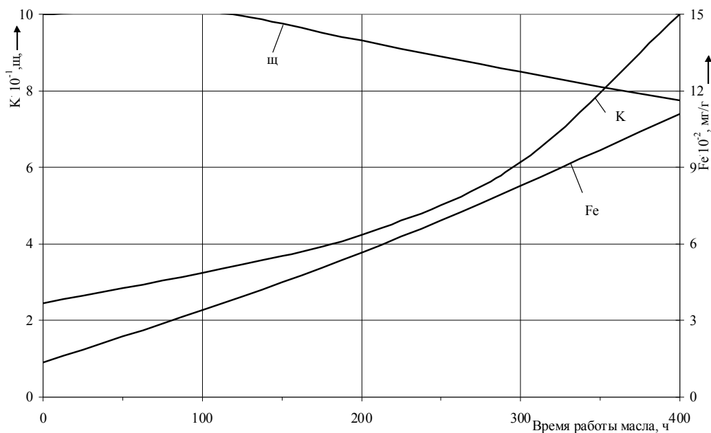
Рис. Изменение служебных свойств моторного масла “МАСТ-ЭКСТРА Дизель”: Щ – щелочность; К – кислотность; Fe – железо
